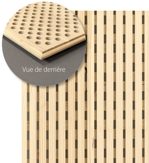
Profil 8/16-16
